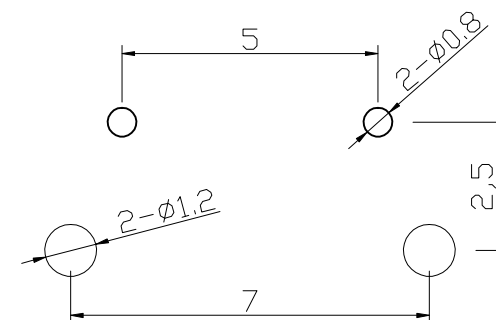
PCB. 焊接图
