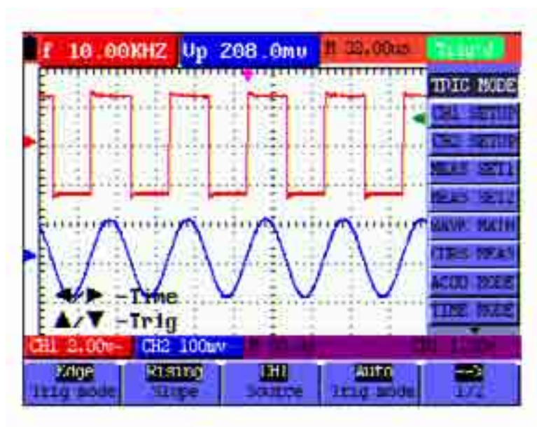
Figure 39: Edge Trigger
