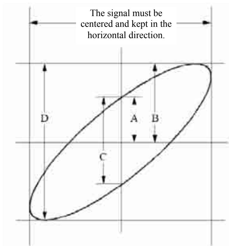
Fig.6-6 Lissajous Graph
